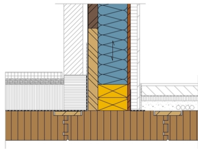
Raccord dalle de plancher - terrasse au mur extérieur
