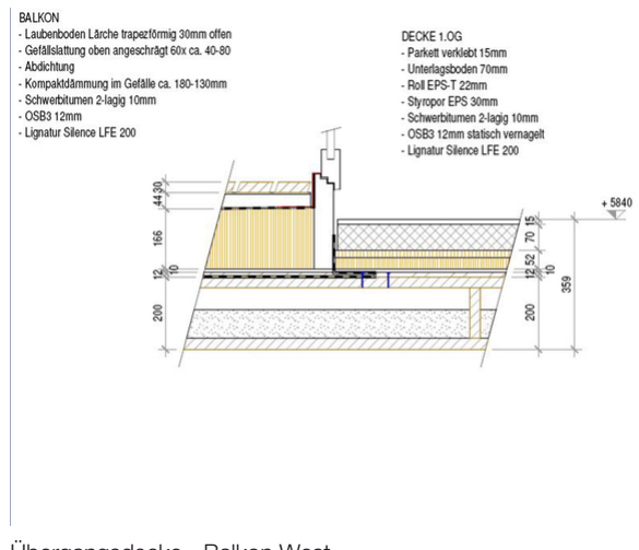
Übergangsdecke - Balkon West
